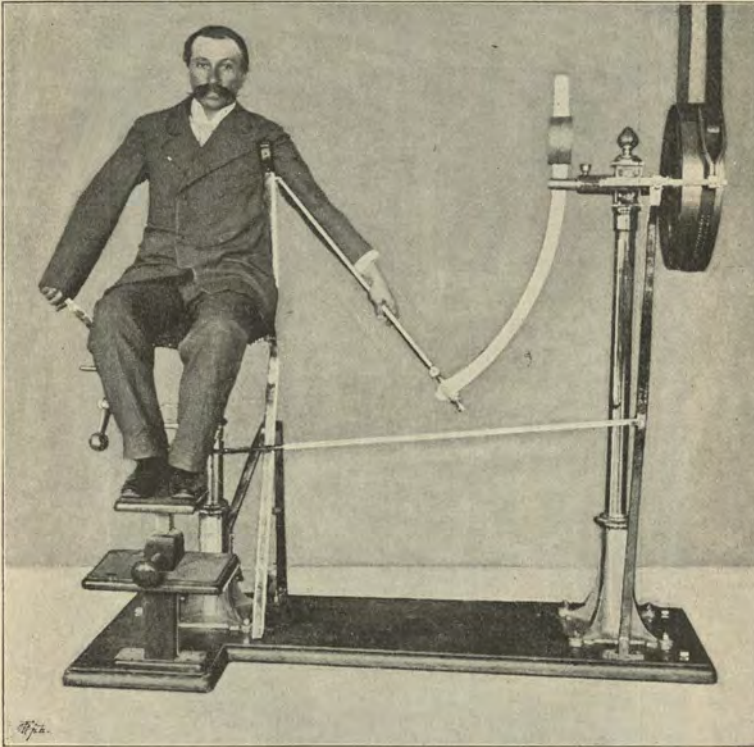
F } O 15 . Arm-Kreisen.
