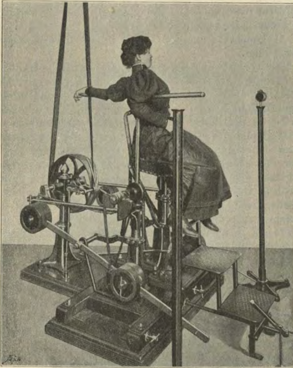
O 11 . Rumpfbiegung. Passiv.
