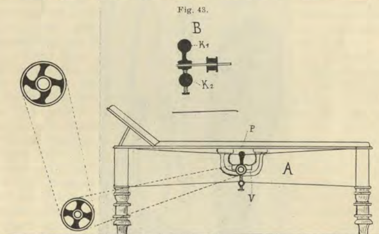
E 2 . Vibrationsbett.
